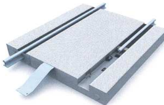
Gleistragplatten mit EBA-Zulassung für Containerterminals, Flug- und Seehäfen, Industrie- und, Gewerbegebiete, etc. im öffentlichen und nicht öffentlichen Bereichen
